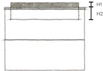
HALBEINBAU-BECKEN
