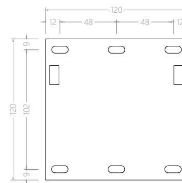
Grundplatte Schwerlastaufhängung
