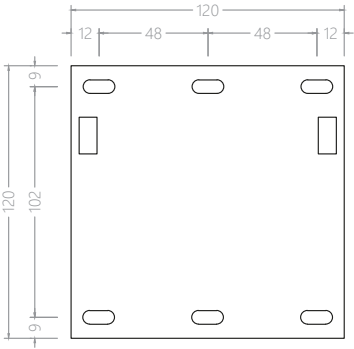
Grundplatte Schwerlastaufhängung
