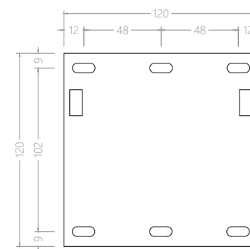
Grundplatte Schwerlastaufhängung
